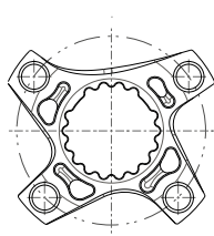
4F. 1X11 76 BCD Ai 5mm CL offset
