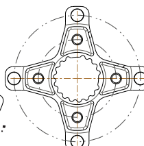
4E. 2X10 64X104 BCD Ai 5mm CL offset
