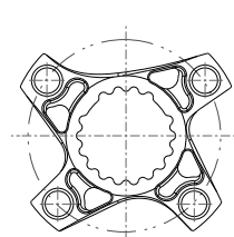
4A. 1X11 76 BCD Ai 5mm CL offset
