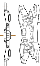
4D. 3X10 64 X 104 BCD
